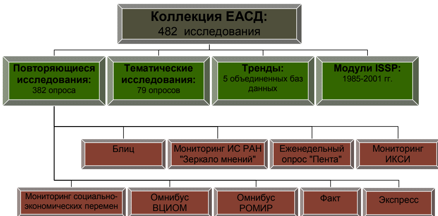
Рис. 3. Структура ЕАСД
